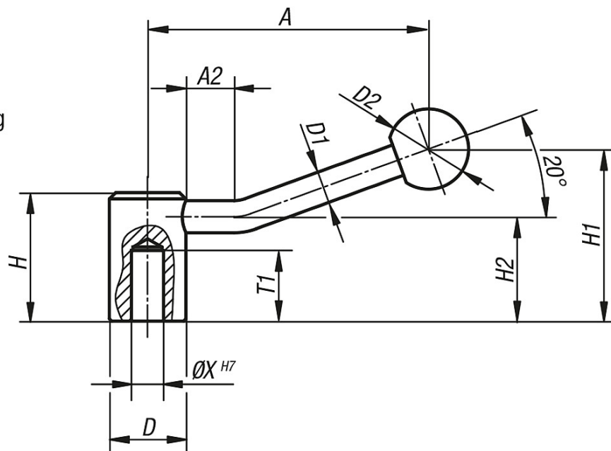
Schaltgriff mit Passbohrung
